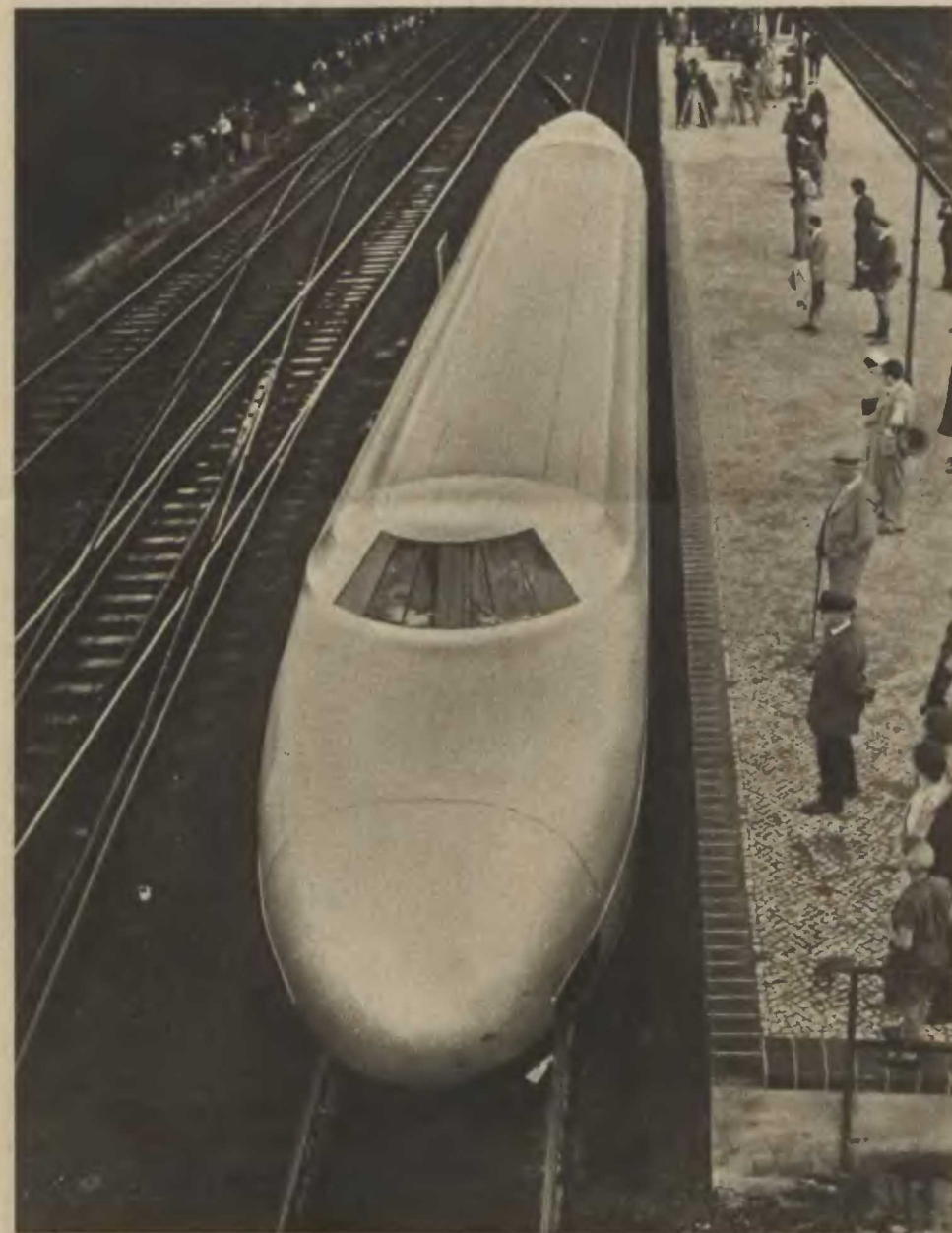
Der „Schienen-Zeppelin“ in Berlin. Das Fahrzeug legte die 257 km lange Strecke von Bergeborf bei Hamburg nach Spandau in einer Stunde 38 Minuten zurück.
