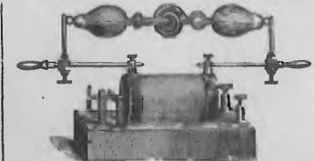
Auf Mahagoni- oder Nussbaumkästen montiert. No. 1 3 mm Funkenlänge Mk. 6,50 " 4 " " " 8,50 " 6 " " " 12,-- " 8 " " " 21,--
