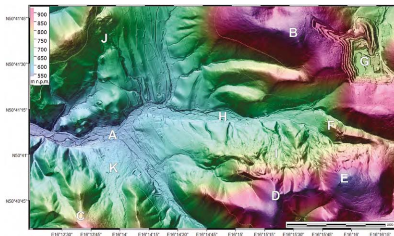
Rys. 1. Wizualizacja NMT powstałego z danych LiDAR, objaśnienia: A – Sokołowsko, B – masyw Bukowca (886 m n.p.m.), C – masyw Garbatki (797 m n.p.m.), D – Włostowa (903 m n.p.m.), E – Suchawa (928 m n.p.m.), F – ruiny zamku Radosno, G – kopalnia melafiru Rybnica Leśna, H – dolina potoku Sokołowiec, I – strefa osuwisk na stokach Włostowej i Suchawy, J – osuwisko na stoku Stożka Małego (745 m n.p.m.), K – akumulacja materiału skalnego w formie rozległego stożka
