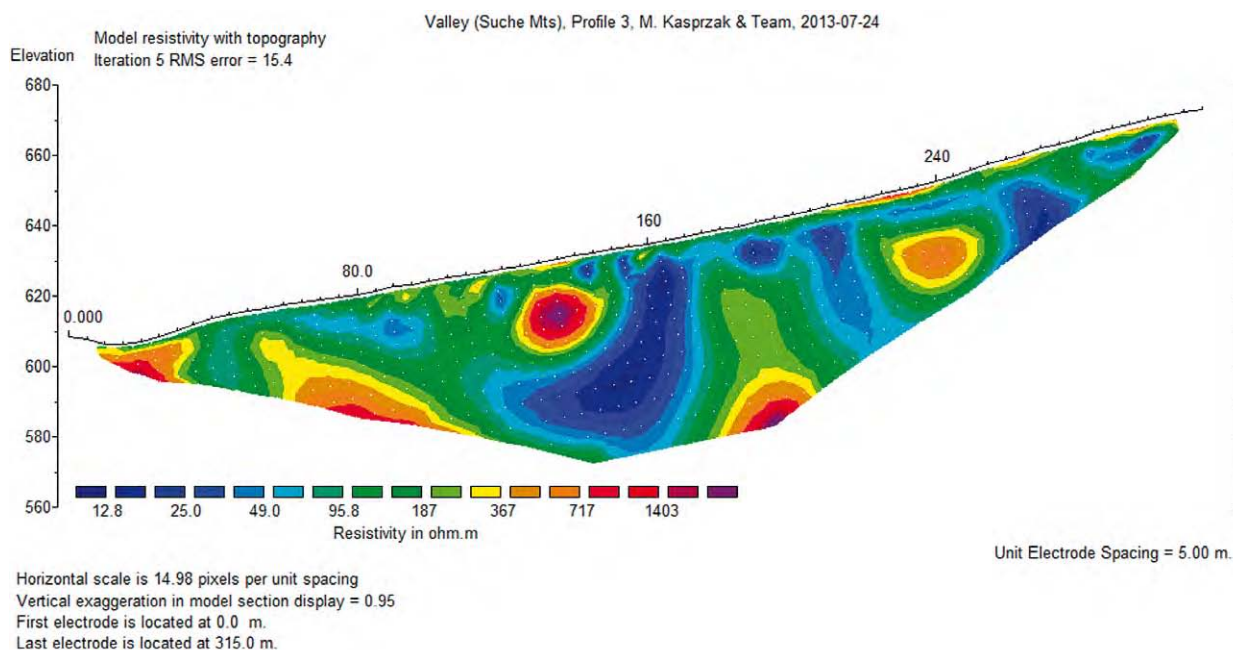
Rys. 2. Tomogram, będący modelem zróżnicowania oporności elektrycznej skał podłoża wzdłuż wyznaczonego profilu o długości 315 m. Poszczególne barwy oznaczają, zgodnie z legendą, oporność elektryczną wyrażoną w omach na metr. Z tomogramu można odczytać zmiany miąższości górnej, przemieszczonej grawitacyjnie warstwy zwietrzelinej skalnej oraz zróżnicowanie struktury głębszego podłoża. Na uzyskany wynik duży wpływ ma system spękań i porowatość skał oraz obecność wody gruntowej
