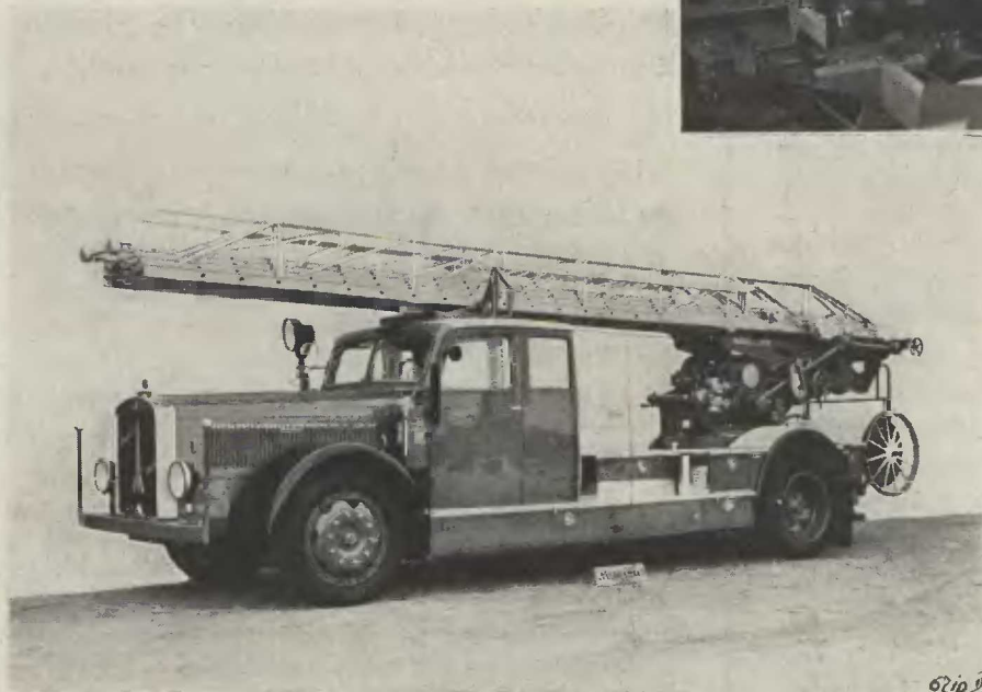
30 m Magirusleiter ein Mustererzeugnis deutscher Hand und Kopfarbeit.
