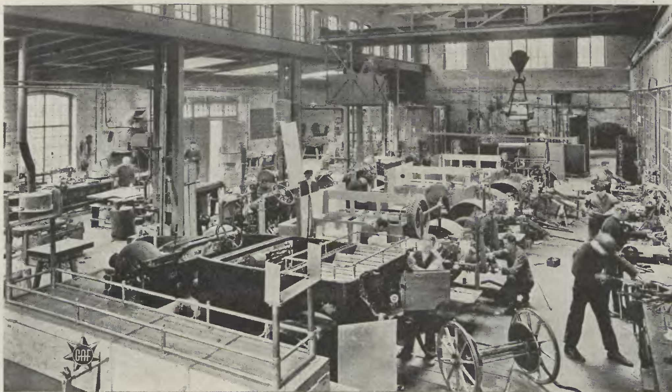
Große Montagehalle für Automobilspritzen
